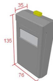
Dimensões Termômetro 1720
